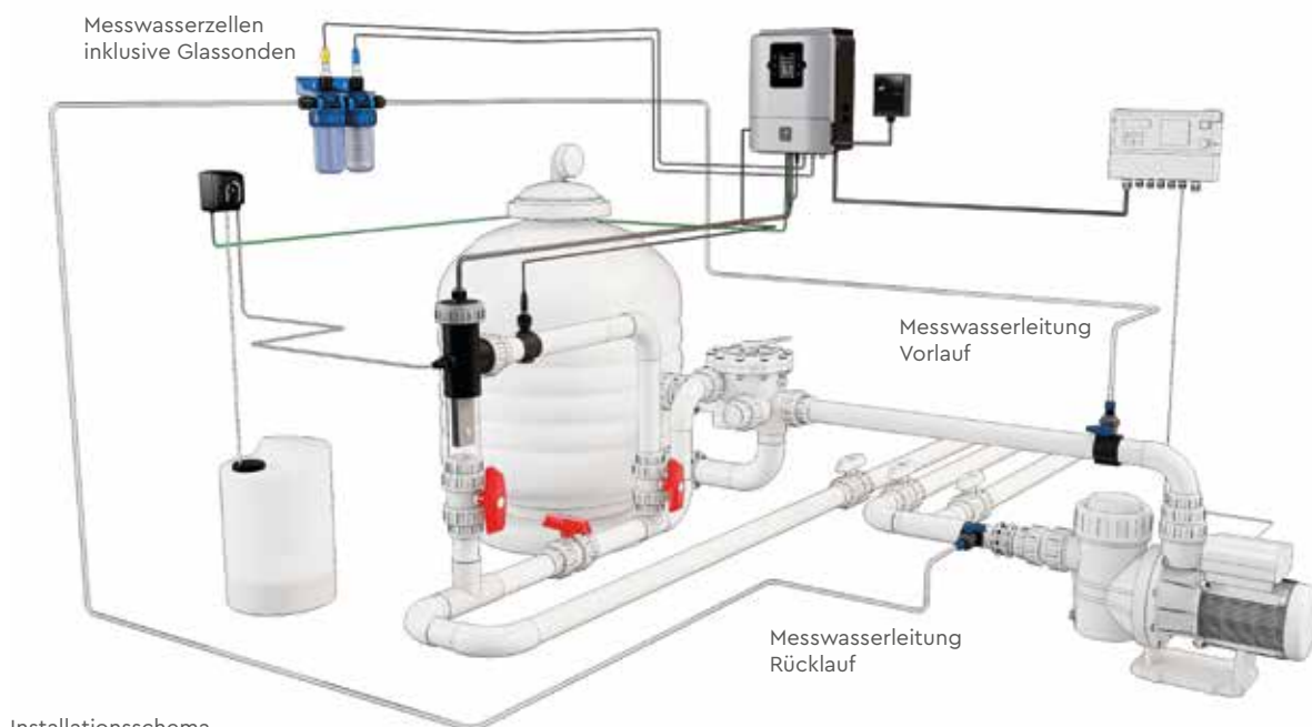
Installationsschema
